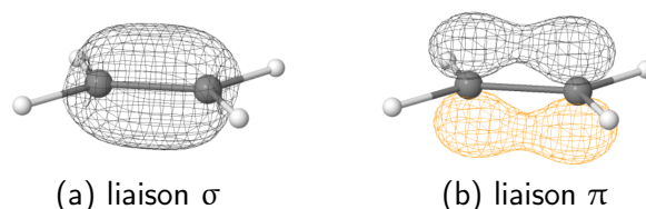
FIGURE 4 – Nature de la liaison éthylénique. (a) Nuage électronique de la liaison \sigma . (b) Nuage électronique de la liaison \pi .
