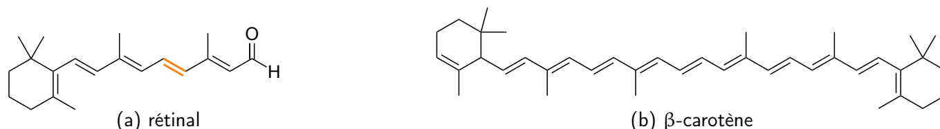
FIGURE 1 – Exemples de dérivés éthyléniques naturels. (a) Rétinal avec la liaison isomérisable marquée en orange. (b) \beta -carotène.
