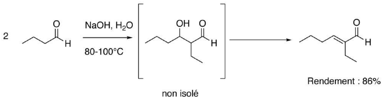
FIGURE 15 – Aldolisation-crotonisation du butanal
