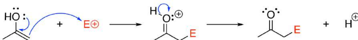
FIGURE 5 – Réaction d'un énol avec un électrophile E^+ : formation d'une cétone \alpha -substituée.
